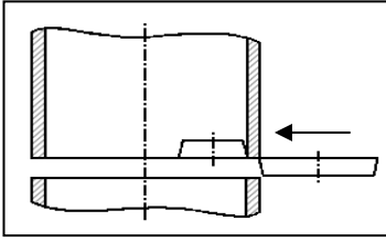
İçe doğru Flanşlama
