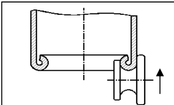
Dikey Kordon Çekme
