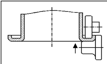
İçe doğru Kıvrırma
