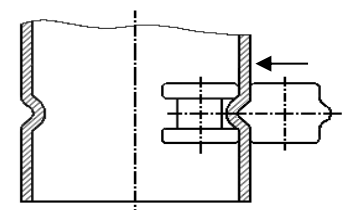
İçten Dikey Kıvrırma
