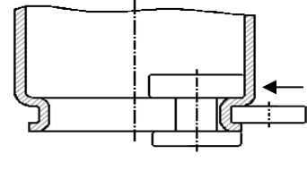
İçe doğru Kordon
