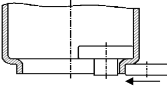
Tankı içe doğru Kıvrırma
