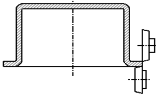
İçe doğru şekil verme
