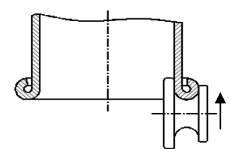
Farklı şekilde Kenetleme
