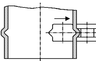
Flanşı Yatay Kıvrırma
